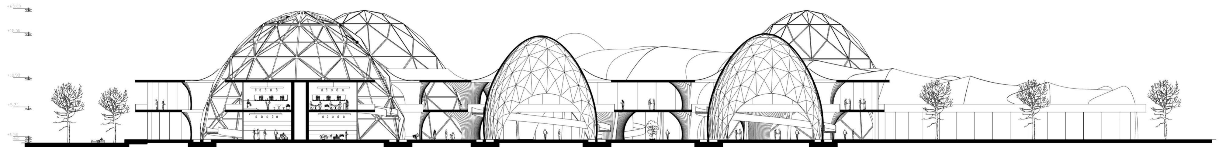
Section A-A
